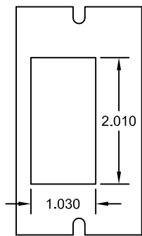
DP009 For Ortronics 2/TJ Bezel
